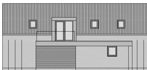
SEVERNÍ POHLED
