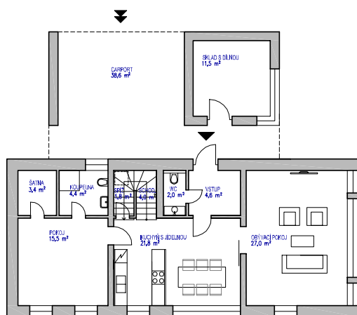
PŮDORYS PŘÍZEMÍ
