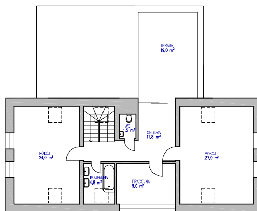
PŮDORYS PODKROVÍ
